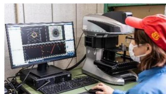
三次元測定機（非接触タイプ）
